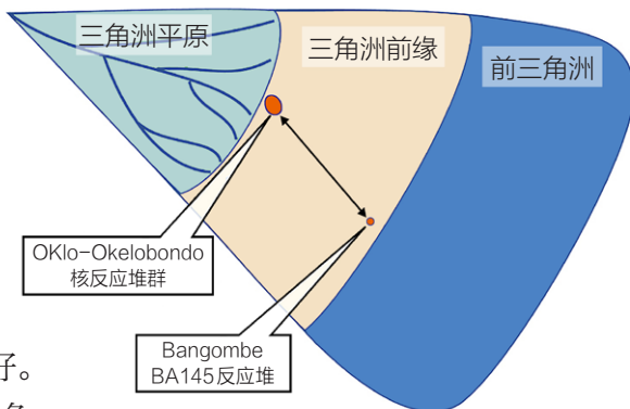
奥克洛露天铀矿 Oklo-Okelobondo 和 Bangombe 核反应堆史前位置
